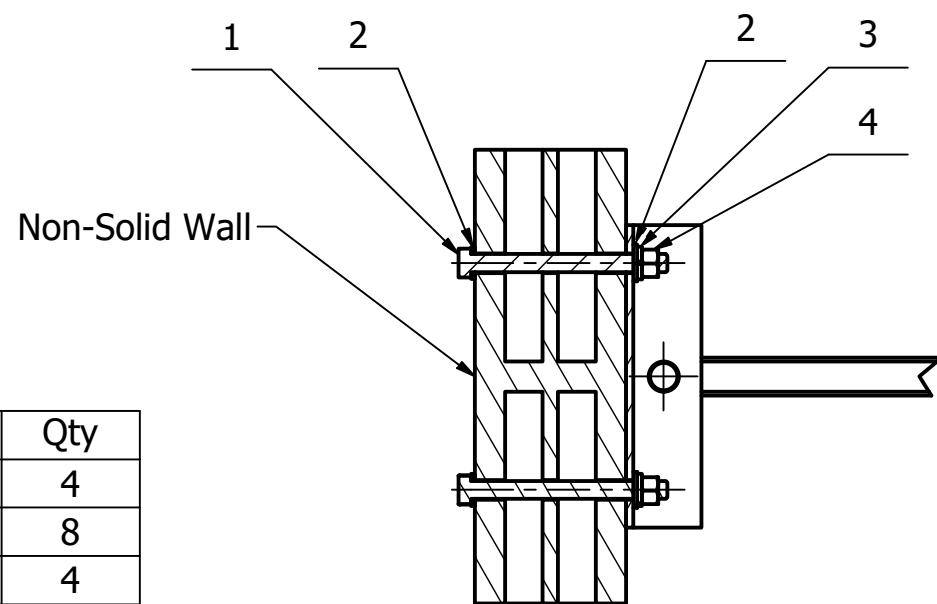
A -A ( 1 : 5 )
