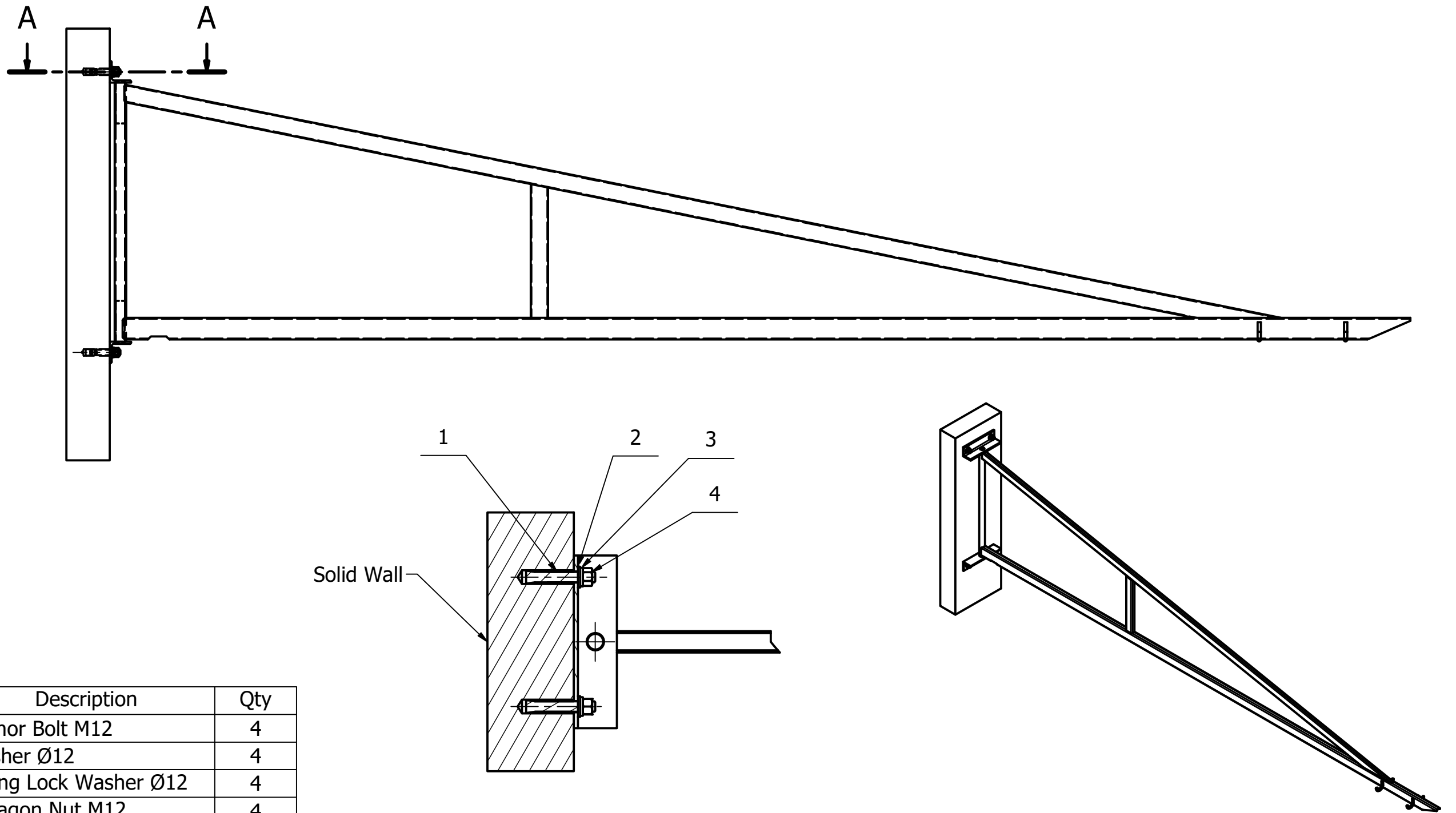
A-A ( 1 : 5 )
